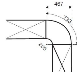
90° Verbindung
